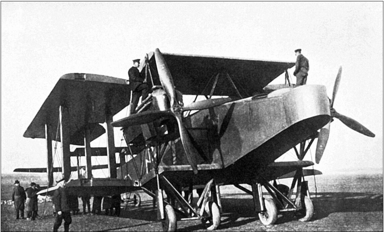
Abb. 53 Auf deutscher Seite notgelandete »Handley Page O/400«. Aufgrund der zunehmenden Verluste traten Moralprobleme auf.
