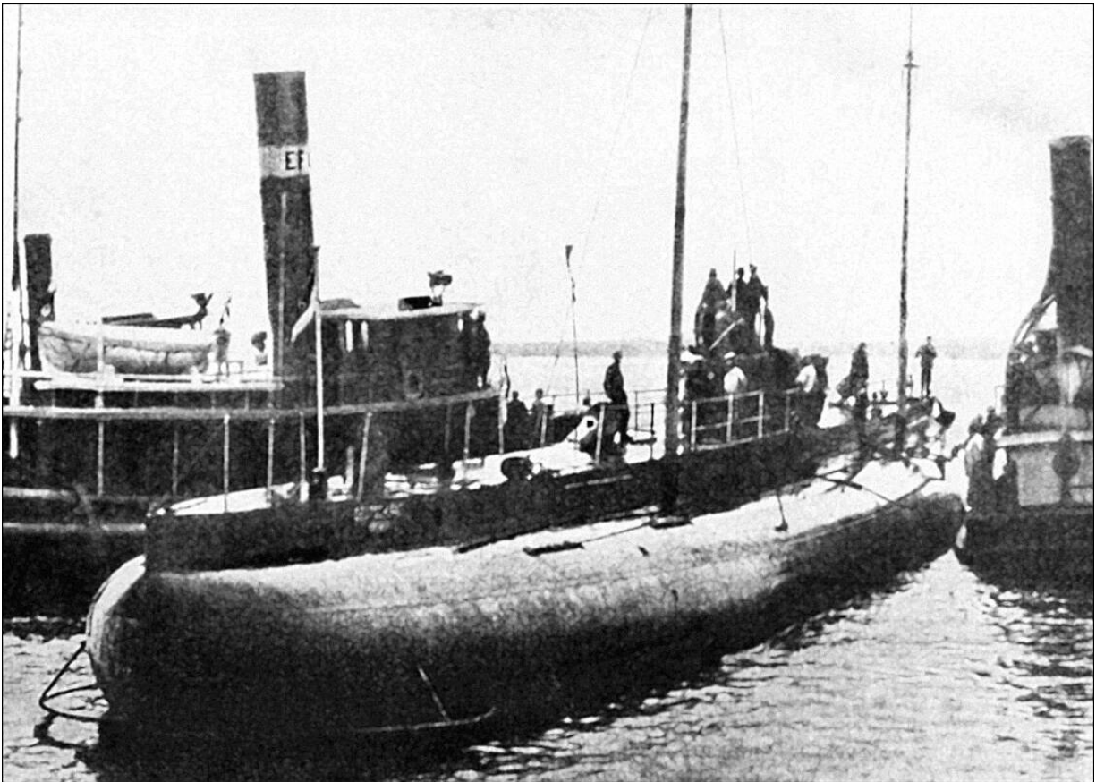
Abb. 24 Handels-U-Boot »U-Deutschland« 1916 in Baltimore. Nach dem Kriegseintritt der USA wurde es zum U-Boot-Kreuzer »U-155« umgebaut und mit zwei 15-cm-Kanonen ausgestattet. 1918 besuchte »U-155« zusammen mit Schwesterschiffen wieder die USA. Dabei versenkten die U-Boot-Kreuzer auf einer Mission 36 alliierte Schiffe, und das trotz schärfster Schutzmaßnahmen der Eskorten.
